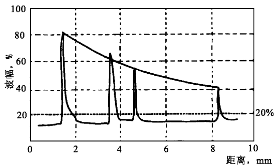
图4 距离一波幅曲线板的范围
