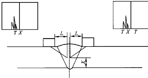
图 F.7 密集缺陷
