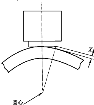
13 探头接触面边缘与管子外表面的间隙示意图
