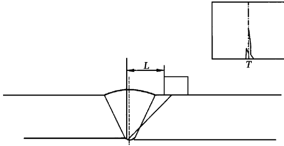
图 F.8 错边
