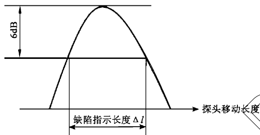
图 10 相对灵敏度法
