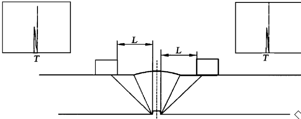
图 F.4 根部未焊透
