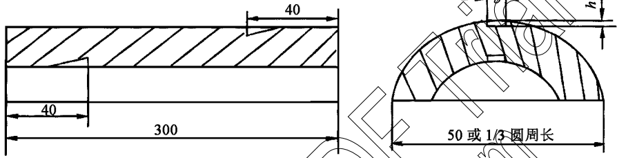
图 18 短槽试块
