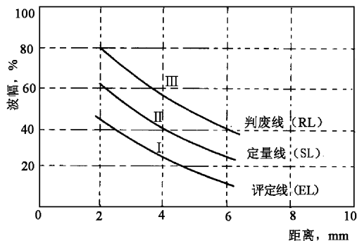
图3 距离一波幅曲线
