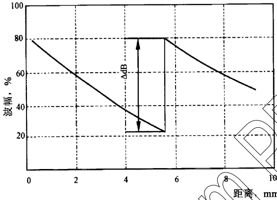
图 5 分段距离—波幅曲线
