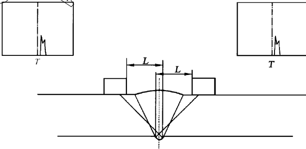
图 F.3 焊瘤
