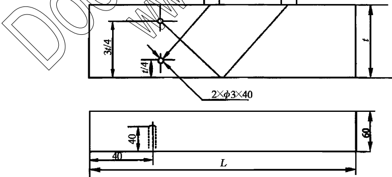
图 E.2 补偿量测定试块
