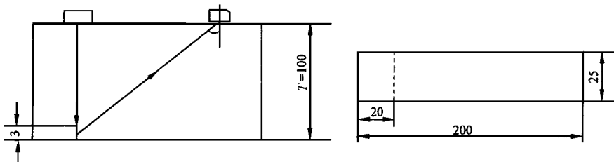
图 C.1 灵敏度调整
