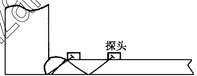
图 16 骑座式角接头
