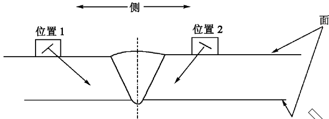
图 2 侧和面
