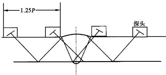
图 15 环向对接接头扫查方法
