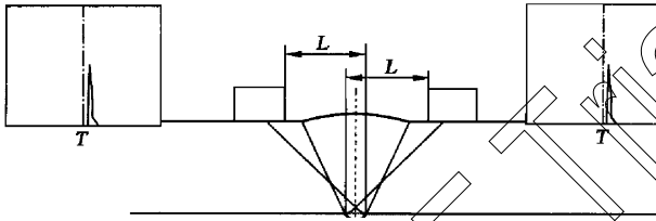
图 F.1 符合要求的焊缝根部
