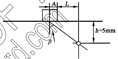
图 I.2 探头折射角测定示意图
