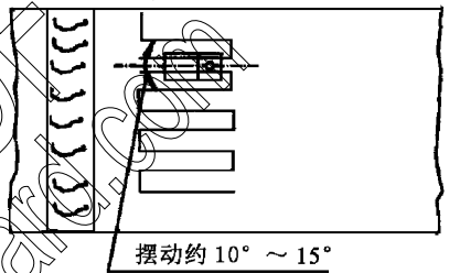
图 6 矩形移动扫查
