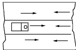
图 8 平行扫查
