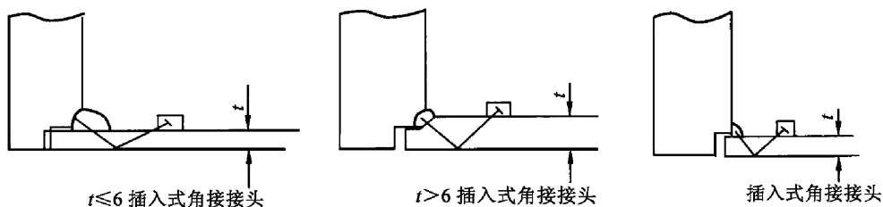
图 17 插入式角接头扫查方法
