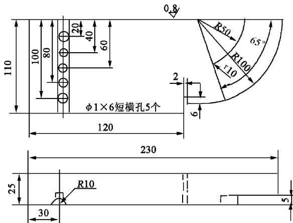
图 1 DRU—I 型试块
