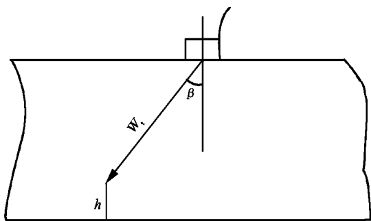
图 4 周向裂纹深度测试示意图
