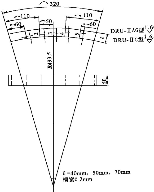
图 2 DRU—II 型试块
