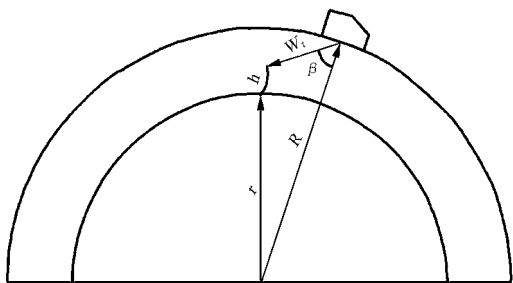
图 3 轴向裂纹深度测试示意图
