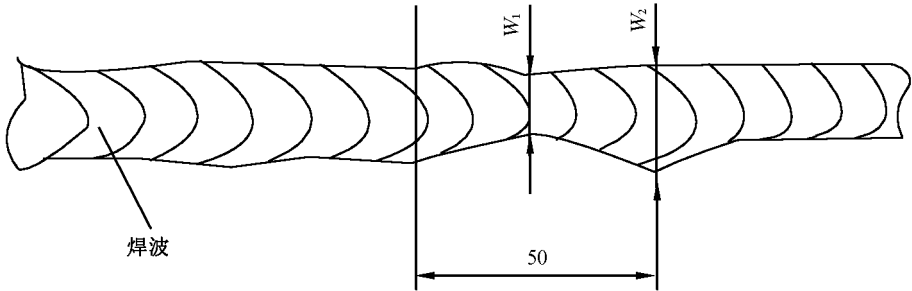
图 5 焊道宽度差
