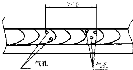
图 10 气孔
