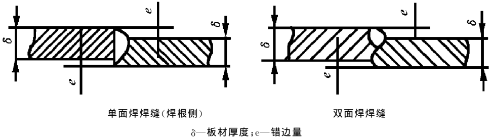
图 7 对接焊缝错边
