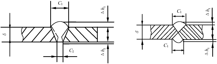
\delta —板材厚度; C_1 —正面焊缝宽度; C_2 —根部焊缝宽度; \Delta h_1 —正面焊缝余高; \Delta h_2 —根部焊缝余高
