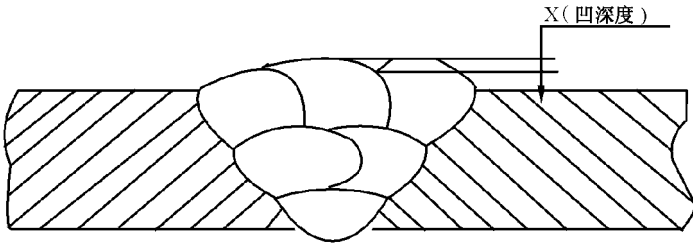
图 4 焊缝表面下凹深度
