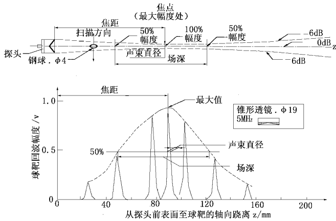
图 11 液浸聚焦探头声束轴线上和横截面声压分布和声束直径
