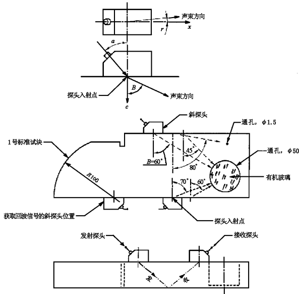
图 4 斜探头接触检测的测试布置
