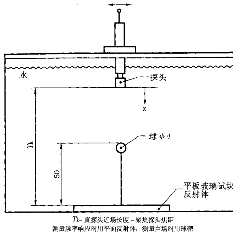
图2 探头置于球靶或平面反射体上方的液浸测试
