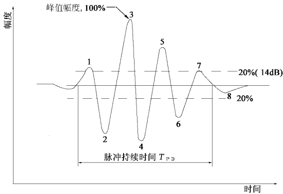
图 5 时域响应
