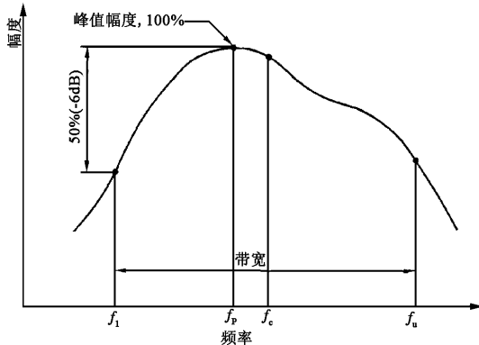
图 6 脉冲回波检测的频率谱
