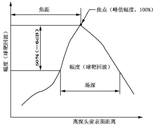
图 10 液浸聚焦探头声束轴线上的声压分布
