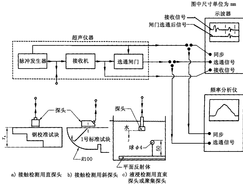
图1 采用电冲击激励的超声脉冲反射法检测的测试装置
