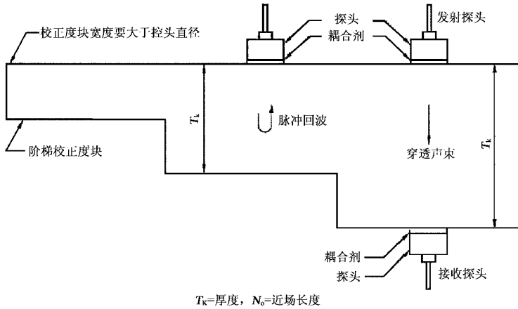
图 3 直探头接触检测的测试布置
