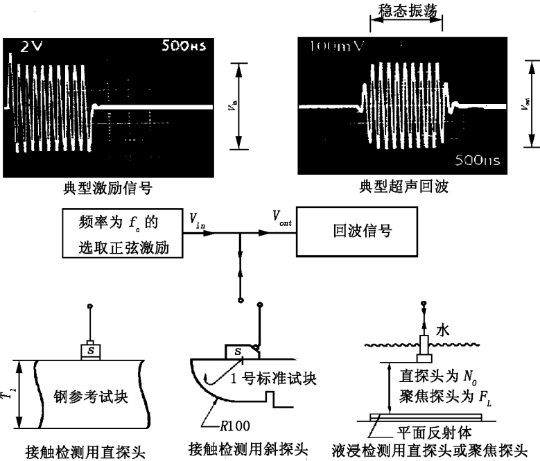
图 12 探头相对灵敏度测量
