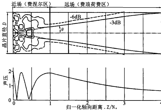
图 9 平探头的自由声场
