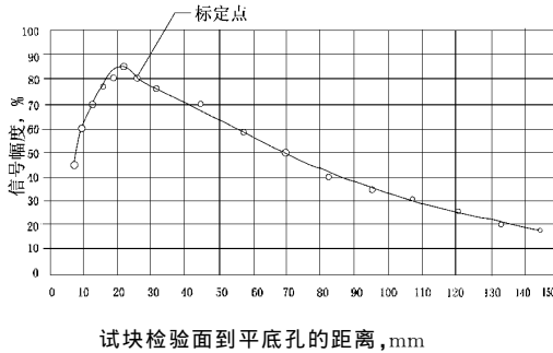
图 4 40CrNi2M. A 钢对比试块距离/幅度超声响应曲线
