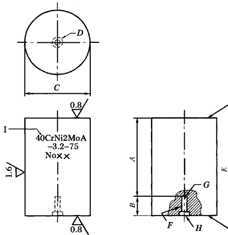
图 1 对比试块的尺寸示意图
