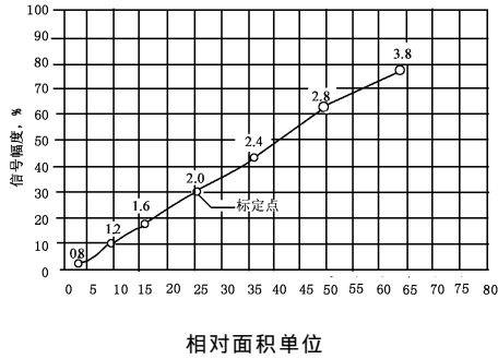
图 3 40CrNi2MoA 钢对比试块面积/幅度曲线
