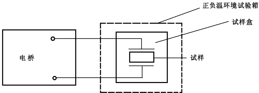
图 3 电桥法测试电路
