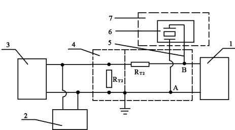
图 1 测 f_s 的线路
